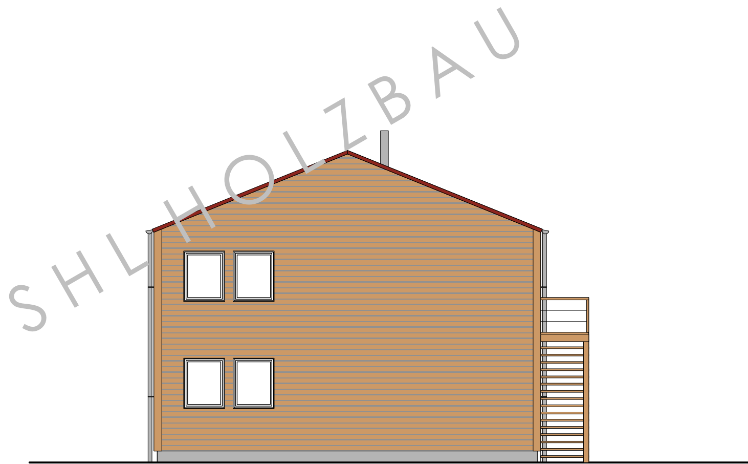
ANSICHT 1
